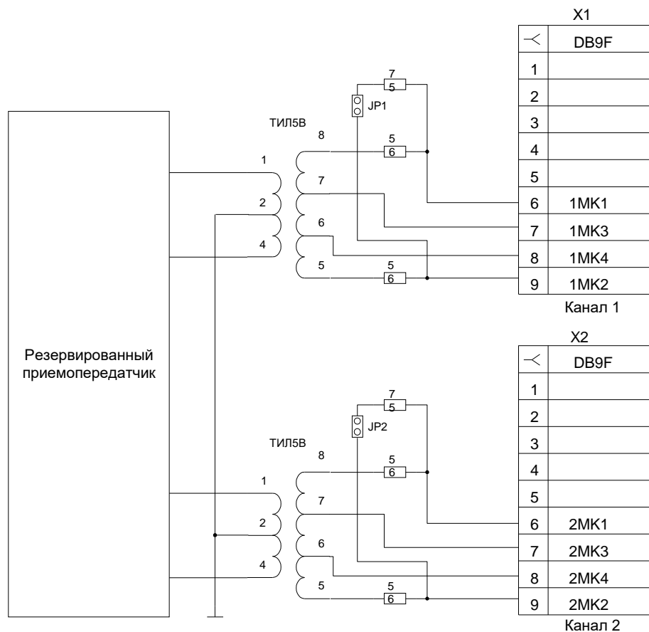
Рис. 8. Подключение устройства к линии передачи информации.
