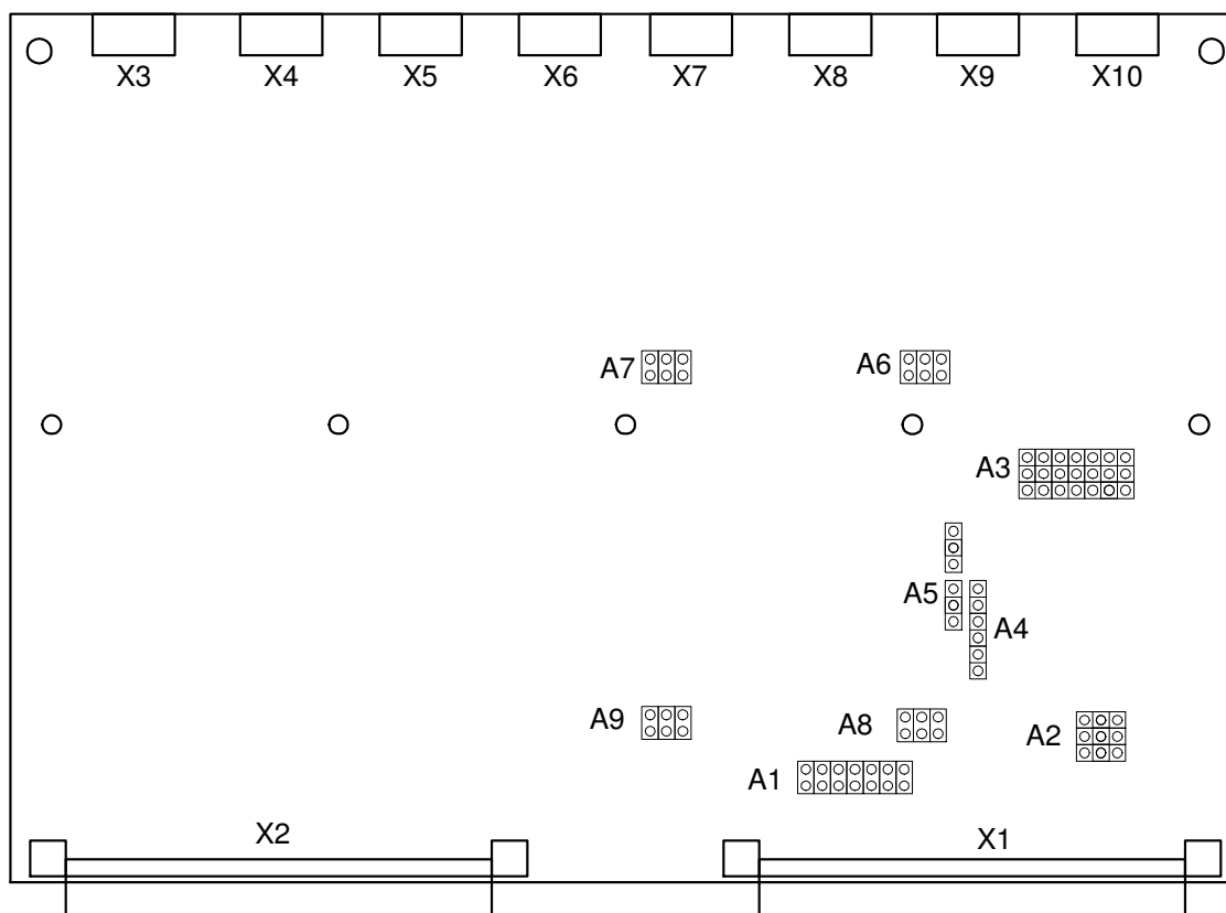
Рис. 5. Условное изображение устройства.
