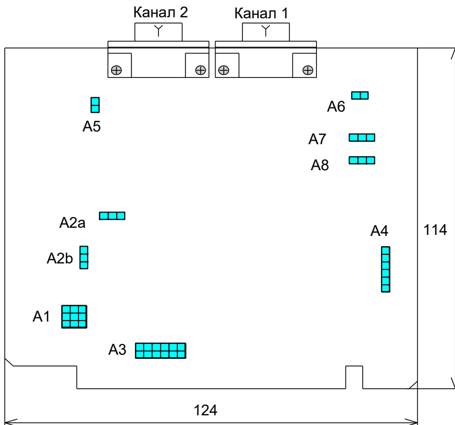
Рис.5б Условное изображение устройства ( вариант Б)
