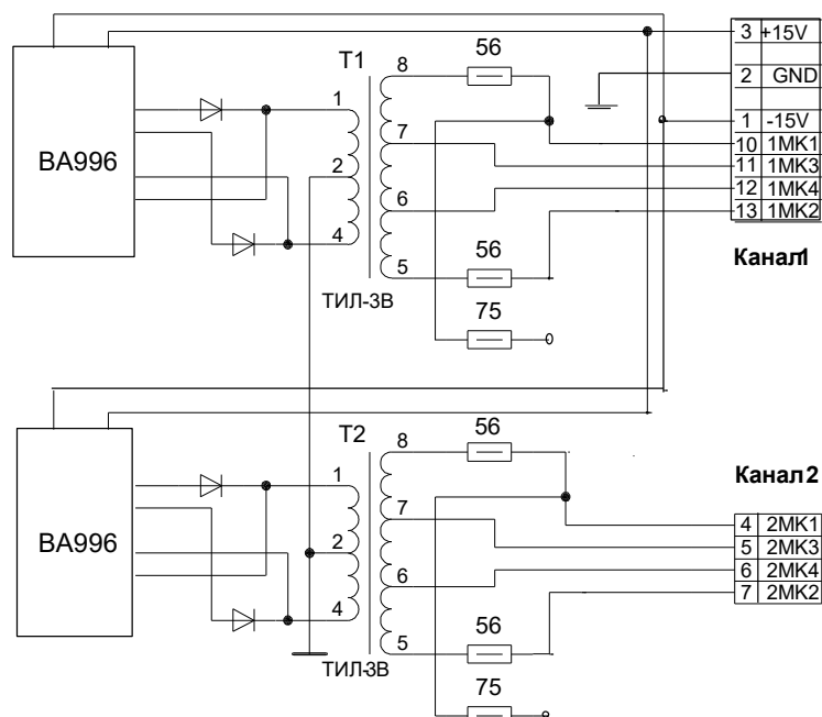
Подключение платы к МК ( вариант А )
