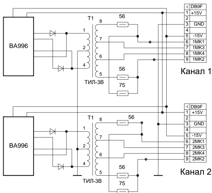
Подключение платы к МК ( вариант Б )
