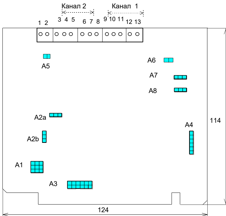
Рис.5а Условное изображение устройства ( вариант А)
