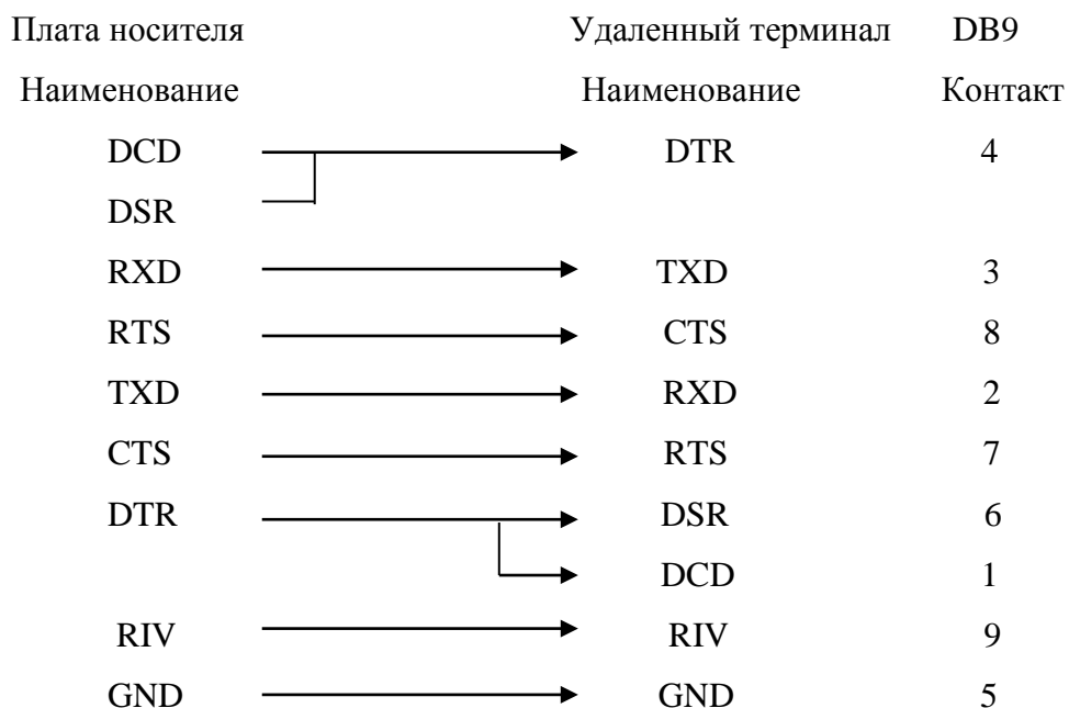
Рисунок 7 Ноль модемный кабель
