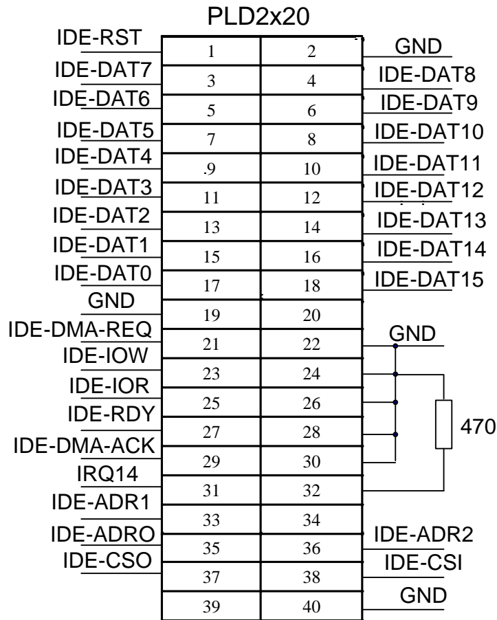
Рисунок 5 Подключение HARD диска
