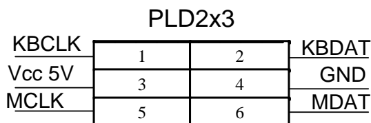
Рисунок 4 Подключение клавиатуры и мыши
