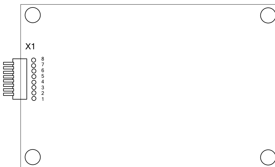
Рисунок 2 Расположение разъемов на плате (верхняя сторона)
